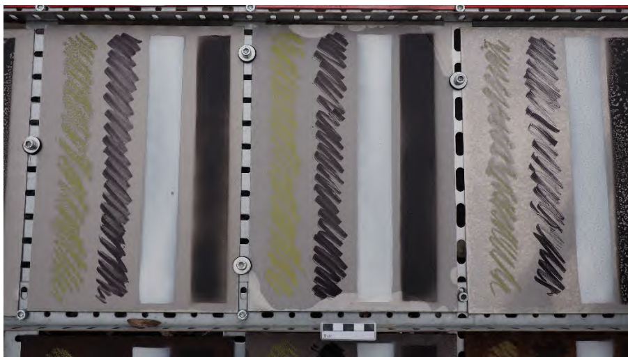
Abb. 18: S4_AGS6 (links), S4_AGS7 (mittig), S4_oAGS (rechts): Abblättern des AGS im Vergleich, hier bei mittlerer Platte S4_AGS7.
