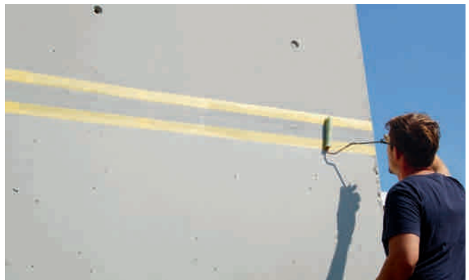
Imprägnierung / Hydrophobierung (z. B. SEMI-Guard) überlappend auf Übergang / Kante aufbringen.
