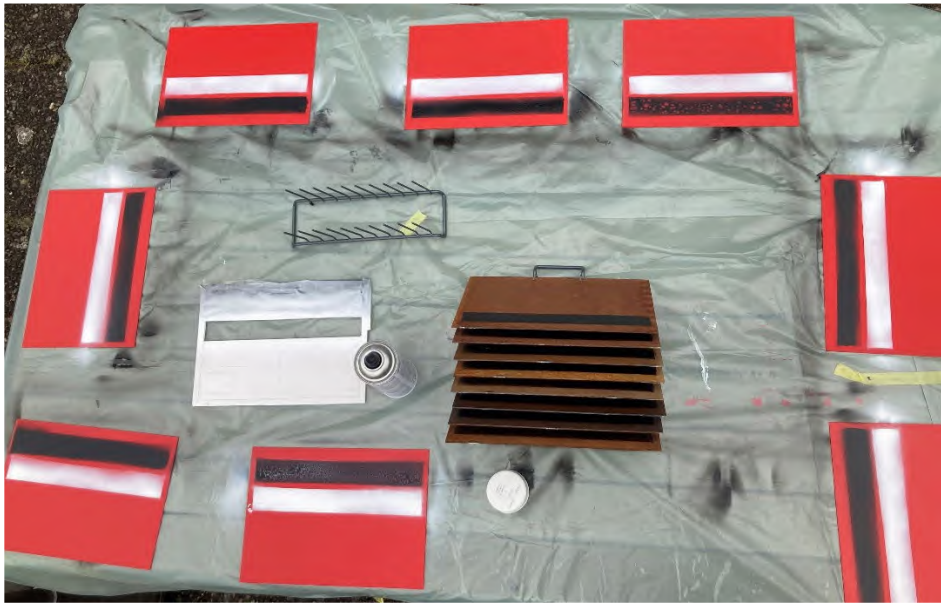
Abb. 13: Auftrag der Sprüh-Graffiti auf die Probeplatten S3 und S5 mit Schablone.
