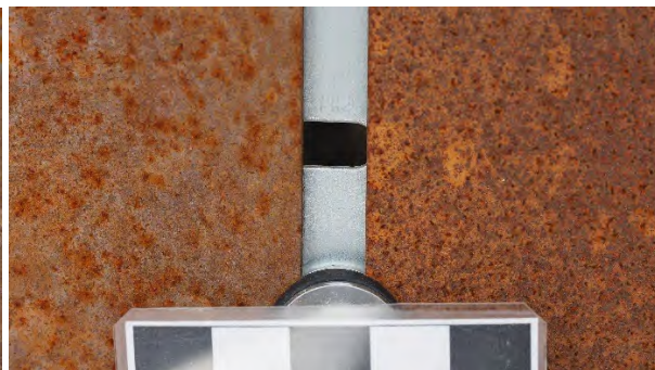
Abb. 12: Platte S5_AGS7 (links) und S5_oAGS (rechts): korrodierte Oberfläche mit Überzug (links), korrodierte Oberfläche ohne Überzug.
