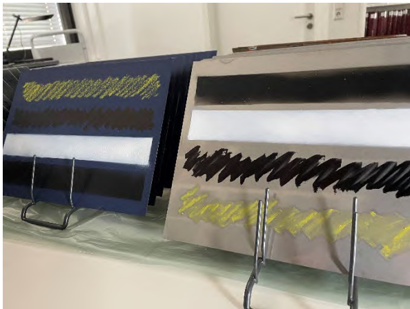
Abb. 14: Prüfkörper mit Graffiti-Medien versehen, vor der erneuten Montage.
