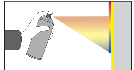
③ Farbanschlag auf permanenten Graffiti-Schutz. Graffiti-Farbe wird an der Oberfläche gehalten. Kein tiefes Eindringen der Farbe in den Untergrund.
