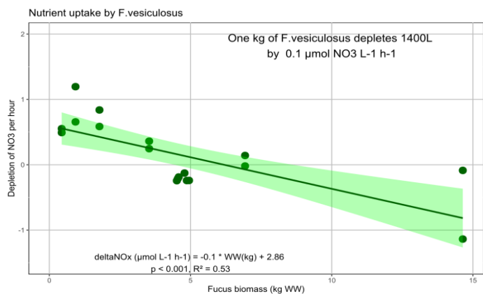
Abb. 7: Nitrat-Abreicherung durch zunehmende Besatzdichte mit Fucus
