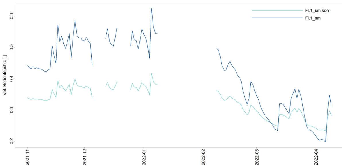
Abbildung 5.1-7: Volumetrische Bodenfeuchte des Forschungsfelds FI.1 im Winterhalbjahr 2021/22 vor (dunkelblau) und nach der Korrektur (hellblau) mit den Gewichtsdaten.
