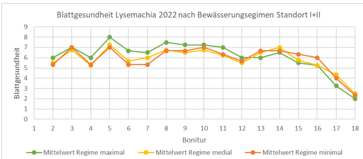
Abbildung 4.3-29: Vergleich der Blattgesundheit von Lysemachia in allen Forschungsfeldern.
