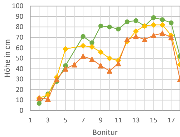
Maximalhöhe Bistorta 2022 nach Feld und Bewässerungsregime Standort II
