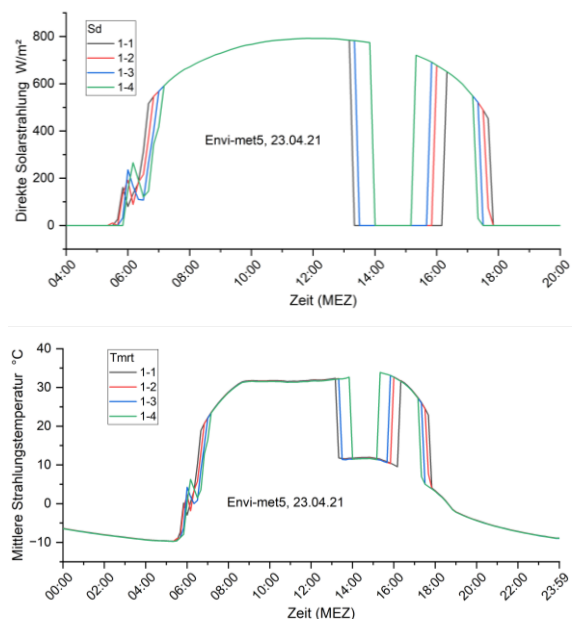
Abbildung 7.3-4: Tagesgang der direkten solaren Einstrahlung und der mittleren Strahlungstemperatur (entspricht der Summe aller Strahlungsströme) auf den Feldern FI-1 bis FI-4.
