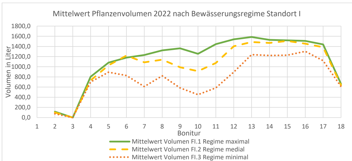
Abbildung 4.3-31: Mittlere Pflanzenvolumina ermittelt aus Bistorta und Geranium in 2022 der Felder FI.1, FI.2 und FI.3.
