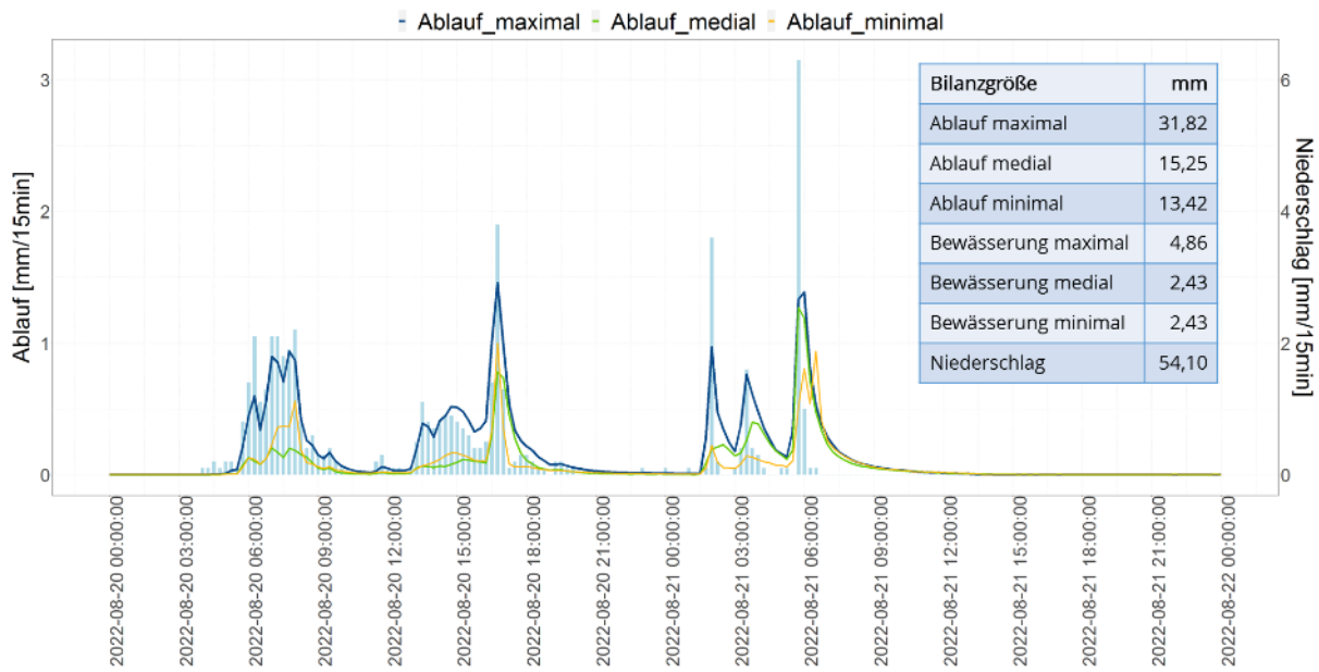
Abbildung 5.1-5: Niederschlag und Abläufe aus den Kippzählermessungen (Forschungsfelder Fl.1 – maximal, Fl.2 – medial, Fl.3 – minimal) für mehrere aufeinander folgende Regenereignisse im Zeitraum 20. – 22.08.2022.
