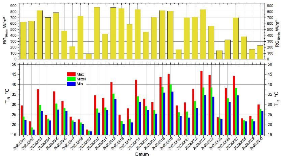
Abbildung 7.2-12: Zusammenhang von Solarstrahlung und Oberflächentemperatur im Juni 2022, 11:00 MEZ, FI.3.
