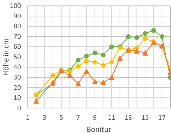
Maximalhöhe Bistorta 2022 nach Feld und Bewässerungsregime Standort I
