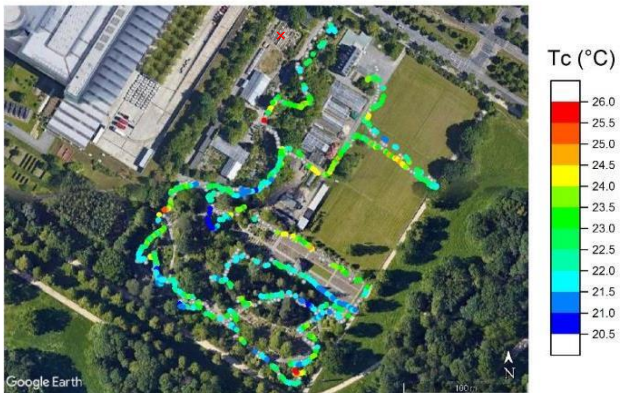
Abbildung 7.3-1: Trendkorrigierte Lufttemperatur während einer Messrunde im Botanischen Garten am 30.03.21, 13:46-14:15 MESZ (Daten aus Projektarbeit P. Volks (s. 3.2.2)): × Lage des Gründachs.
