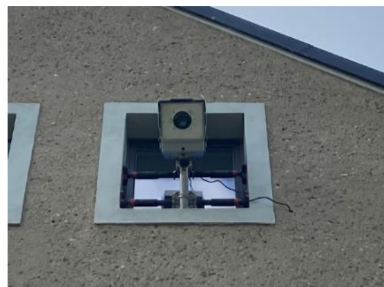
Abbildung 7.1-3: Position und Ausrichtung des Infrarotsensors am Verwaltungsgebäude des Botanischen Gartens. Das Messfeld entspricht etwa dem Fotoausschnitt in Abbildung 7-4 (Foto: V. Goldberg, 11.08.2021 und 07.09.2022).
