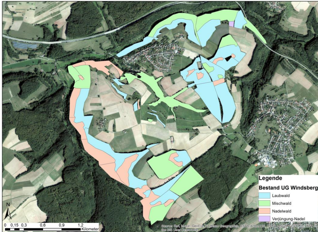
Abbildung 15 Die am Tag von der Drohne durchgeführte Kartierung der Waldhabitate in dem UG Windsberg gibt Aufschluss über die Flächenanteile, welche eine verstärkte Übersehrate abbilden und somit der Korrektur unterliegen. Hier in der Karte wurde zwischen Laub-, Nadel- und Mischwald und Verjüngung Nadelwald unterschieden.
