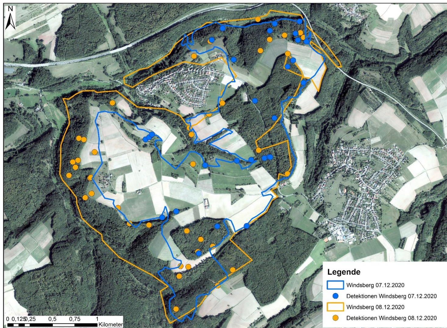
Abbildung 13 Die Erfassungen des UG Windsberg fanden am 07. – und 08.12.2020 statt. Die Befliegungsfläche unterschied sich um ca. 179 ha, da am 07.12.2020 ca. 357 h und in der darauffolgenden Nacht 536 ha erfasst wurde. Das UG befindet sich außerhalb des Pfälzerwaldes – im südwestlichen Bereich.
