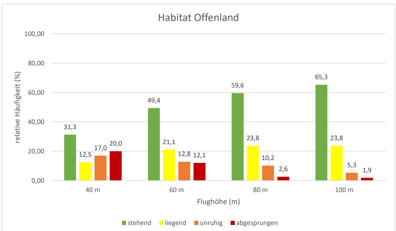
Anhang Abbildung 3 Dargestellt ist das nächtliche Verhalten der beobachteten Rehe in Abhängigkeit der Flughöhe der Drohne in Offenland Habitaten.
