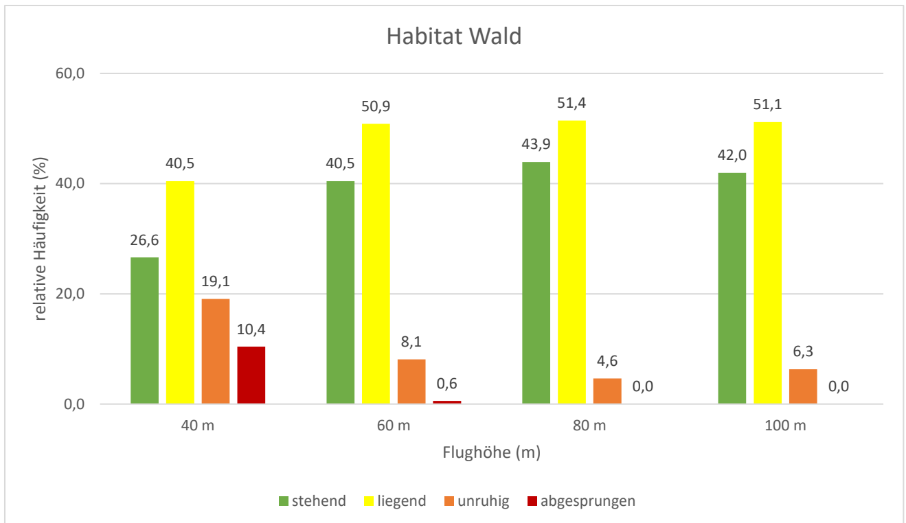
Anhang Abbildung 2 Dargestellt ist das nächtliche Verhalten der beobachteten Rehe in Abhängigkeit der Flughöhe der Drohne in bewaldeten Flächen.
