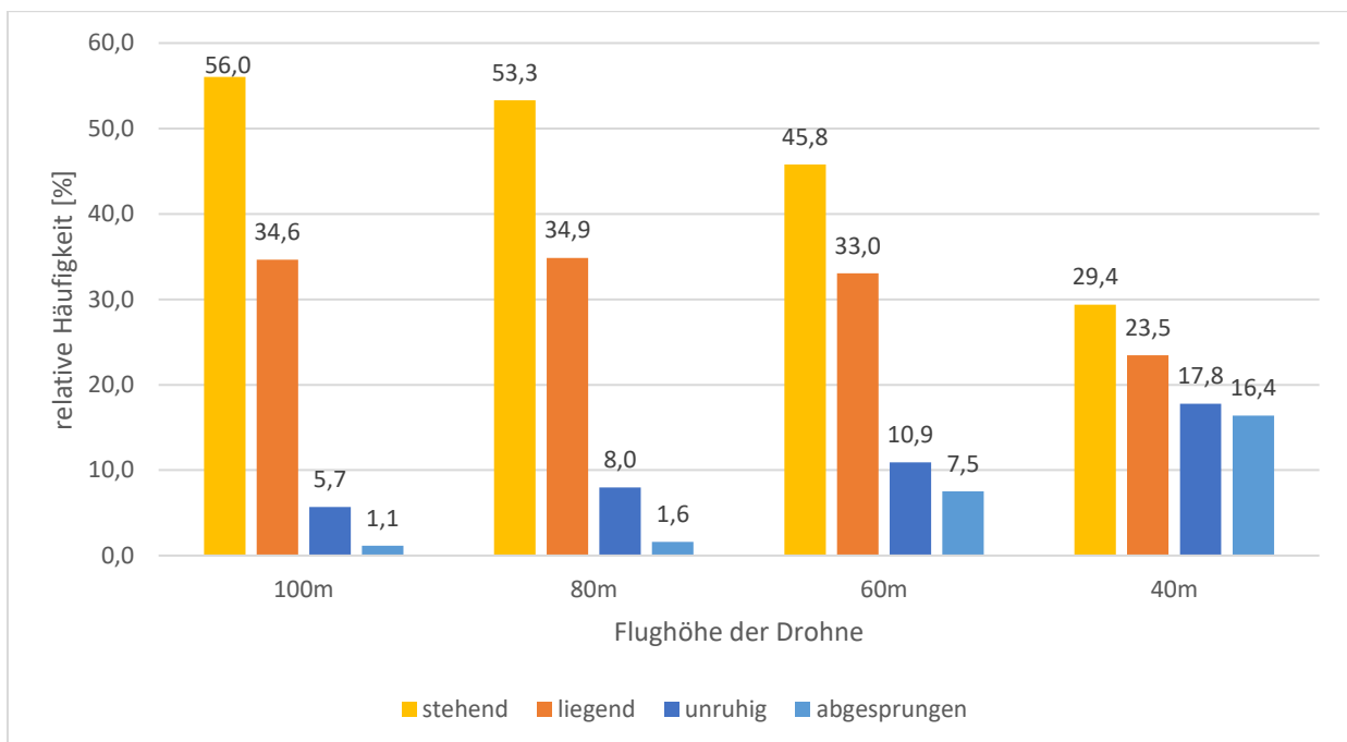
Abbildung 10 Dargestellt ist das nächtliche Verhalten der beobachteten Rehe in Abhängigkeit der Flughöhe der Drohne in Wald und Offenlandgebieten (nicht differenziert).
