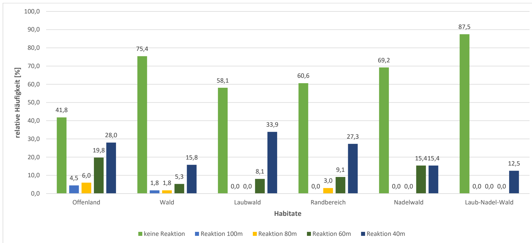
Anhang Abbildung 1 Relative Häufigkeitsverteilung der Störversuche in Relation zu Habitat und Drohnenflughöhe für Rehwild im und in der Umgebung des Pfälzerwaldes. Reaktionen unterteilen sich in „keine Reaktion“ und Reaktion bei einer Drohnen-Flughöhen von 100m bis 40m
