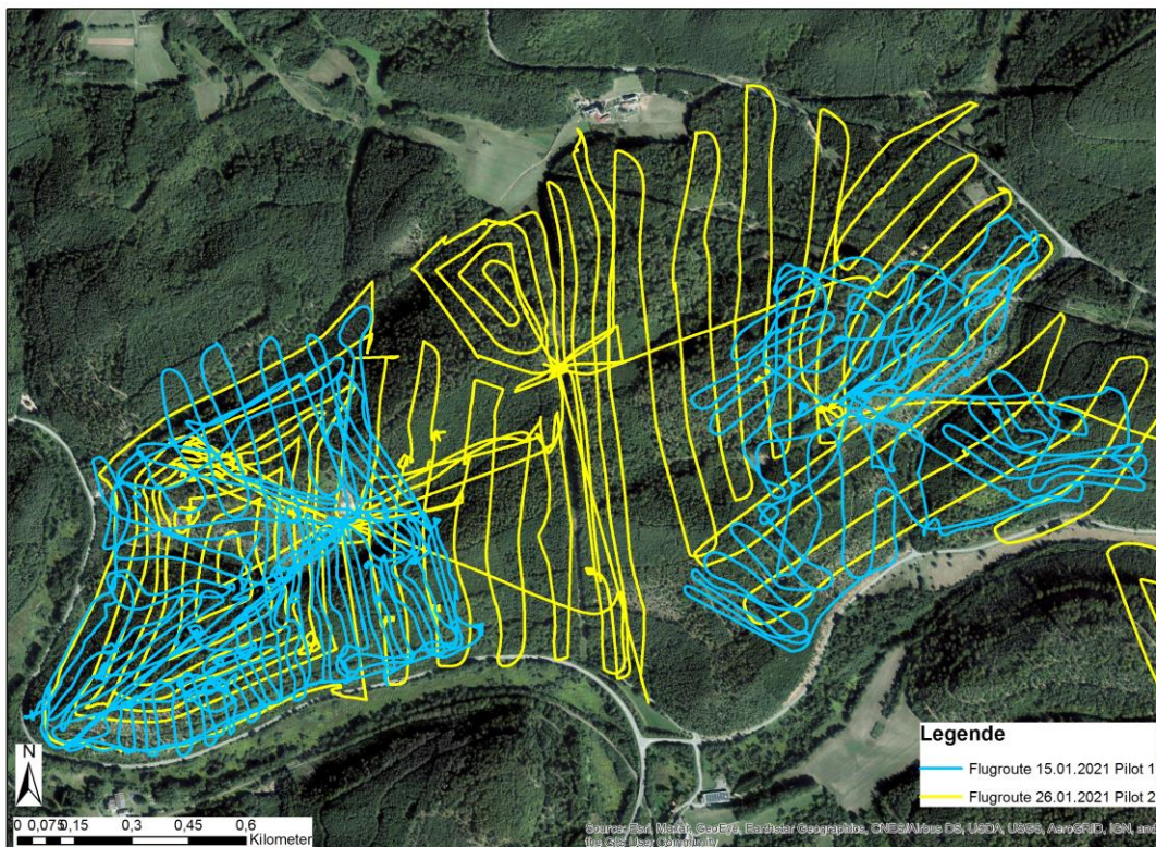
Abbildung 16 Flugroutendichte von zwei Drohnenpiloten am Beispiel des UG Hinterweidenthal I. Die Flugroutendichte pro geflogenen 100 ha Revierfläche kann sich von Pilot zu Pilot stark unterscheiden ( Tabelle 4 ).
