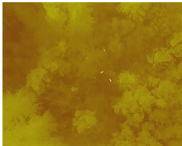
Abbildung 6 Erfassung von Rehwild in einer bewaldeten Fläche auf einer Drohnen-Flughöhe von ca. 80 m. © FAWF Landesforsten RLP
