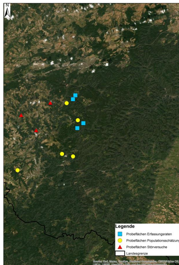
Abbildung 4 Übersicht über die Untersuchungsflächen im Pfälzerwald und dessen unmittelbarer Umgebung. Unterschieden wird in der Übersicht in Probestflächen für Störversuche, Erfassungsraten und Populationschätzungen. Diese Versuche wurden in dem Zeitraum von Oktober 2019 – April 2021 durchgeführt.
