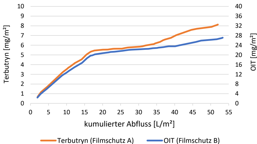
Abbildung 4: Kumulierte Emission vs. kumulierten Abfluss für Terbutryn (konventionelles Produkt, Probefläche 2) und OIT (neues Produkt, Probefläche 4) im Fassadenabfluss der Versuchsflächen (Werte pro m 2 ).
