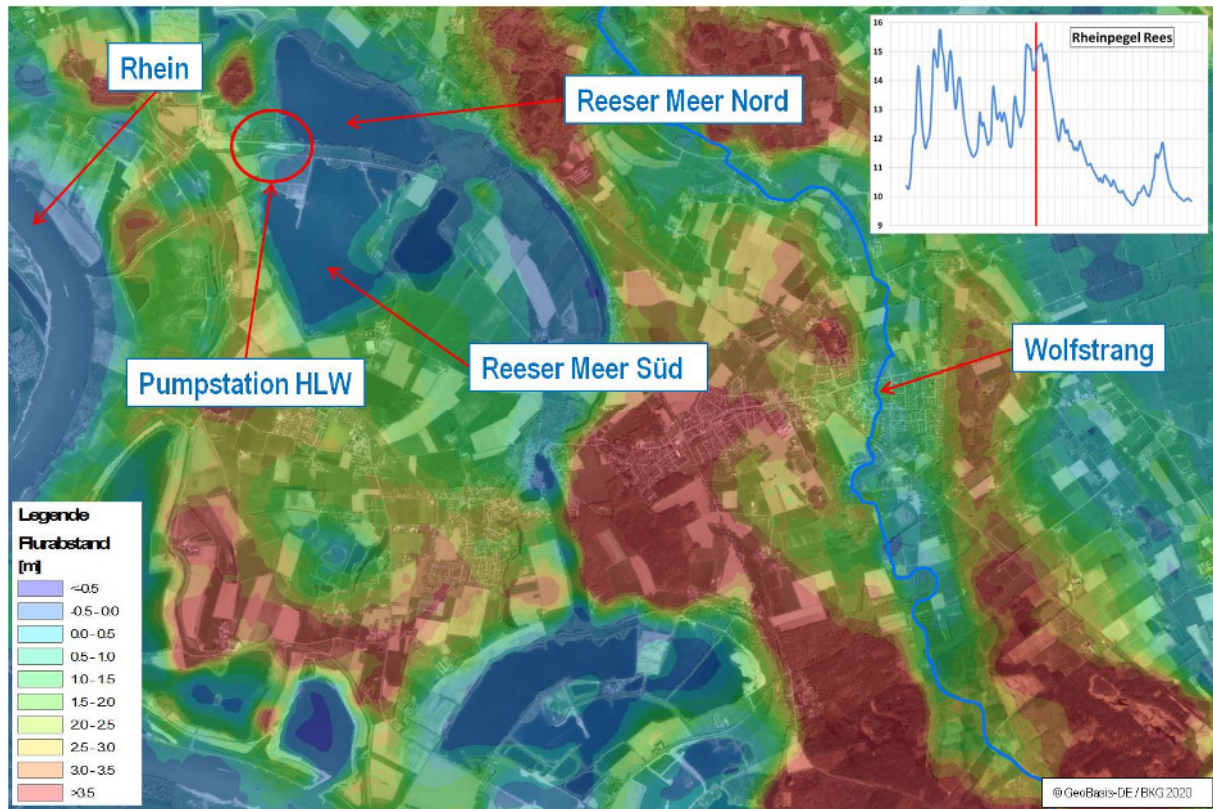
Abbildung 6.9: Flurabstände im Deichhinterland im Bereich der Haffenschen Landwehr (HLW) und Wasser- tandsganglinie für den Rheinpegel Rees
