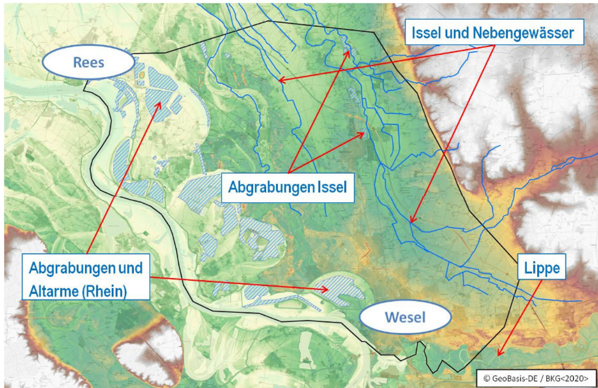
Abbildung 5.2: Gewässer im IJssel 2D-Hydraulikmodell und Abgrabungen / Altarme am Rhein
