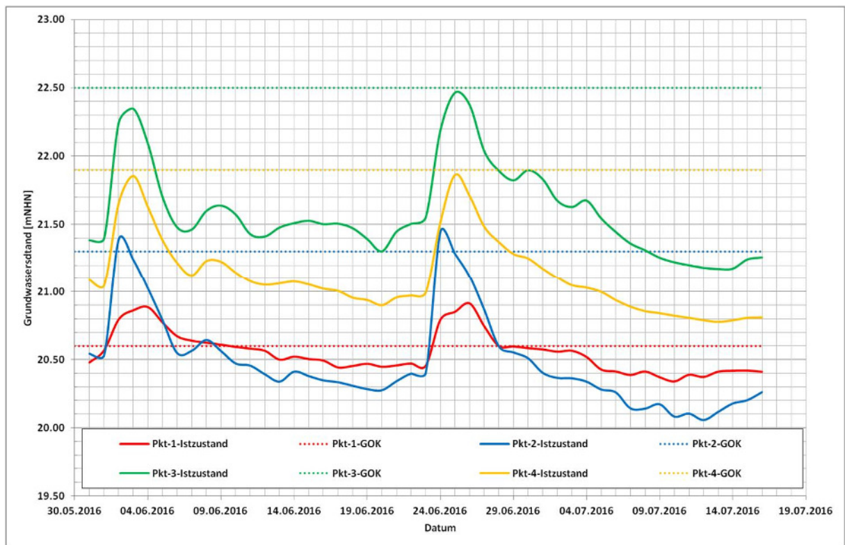
Abbildung 6.7: Grundwasserganglinien und Geländeoberkanten für die Grundwasser-Messpunkte entlang der Issele
