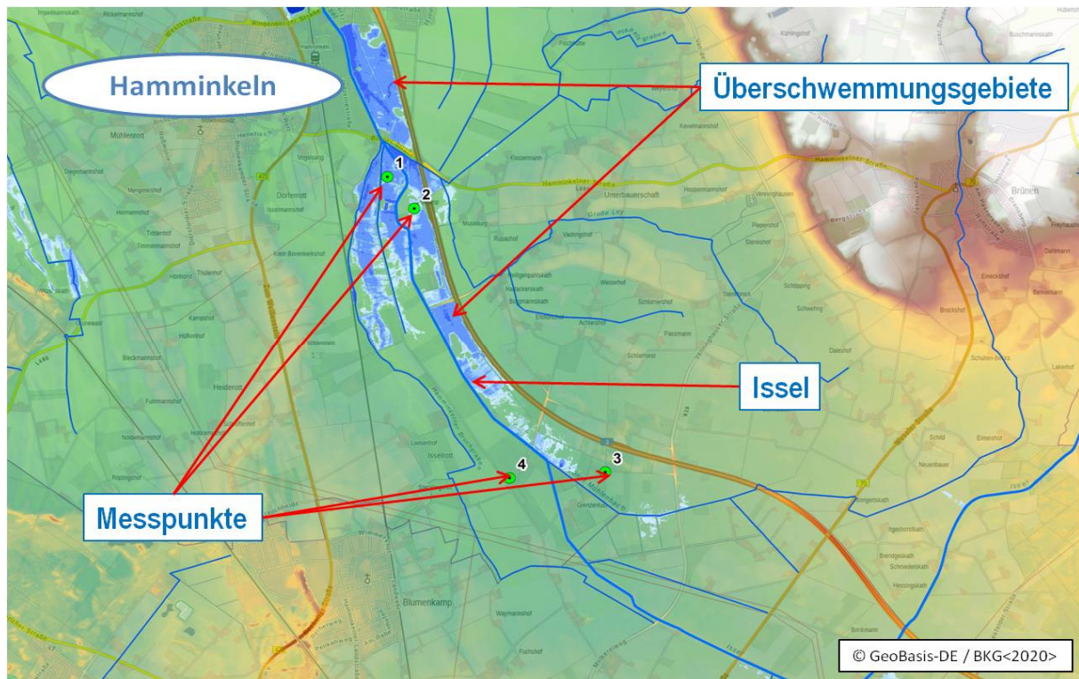
Abbildung 7.4: Überschwemmungsgebiete oberhalb von Hamminkeln im Planzustand und Lage der Grundwasser-Messpunkte entlang der Isse l
