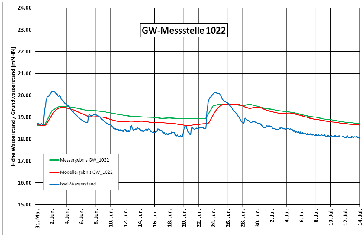
Abbildung 5.14: Gemessene und berechnete Grundwasserstände für die Messstelle GW_1022 sowie der Issel-Wasserstand im Nahbereich der Messstelle
