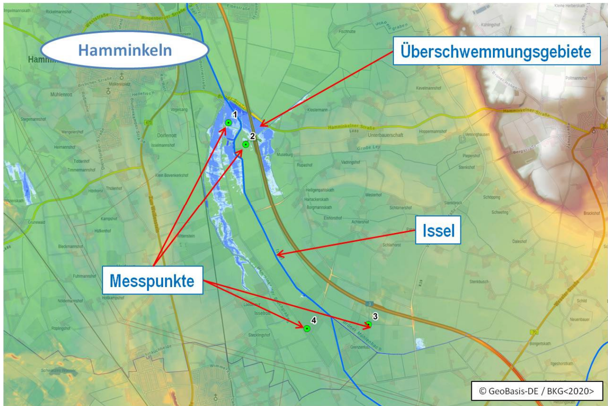
Abbildung 6.6: Überschwemmungsgebiete oberhalb von Hamminkeln und Lage der Grundwasser-Messpunkte entlang der Issele
