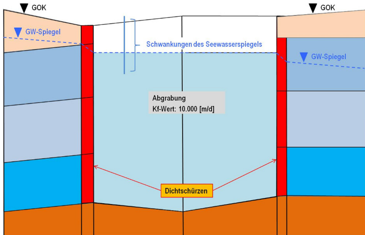
Abbildung 5.9: Schematische Darstellung einer Abgrabung im Grundwassermodell
