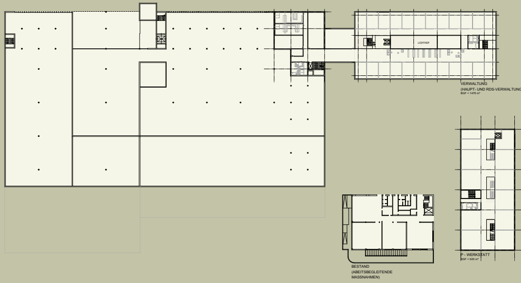
grundriss obergeschoss1 m1zu500
