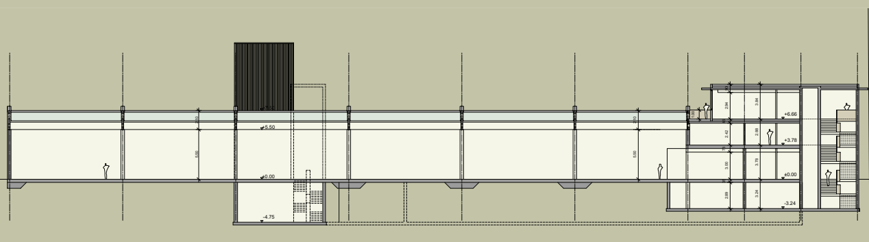
längsschnitt m1zu200 bauberschnitt 1
