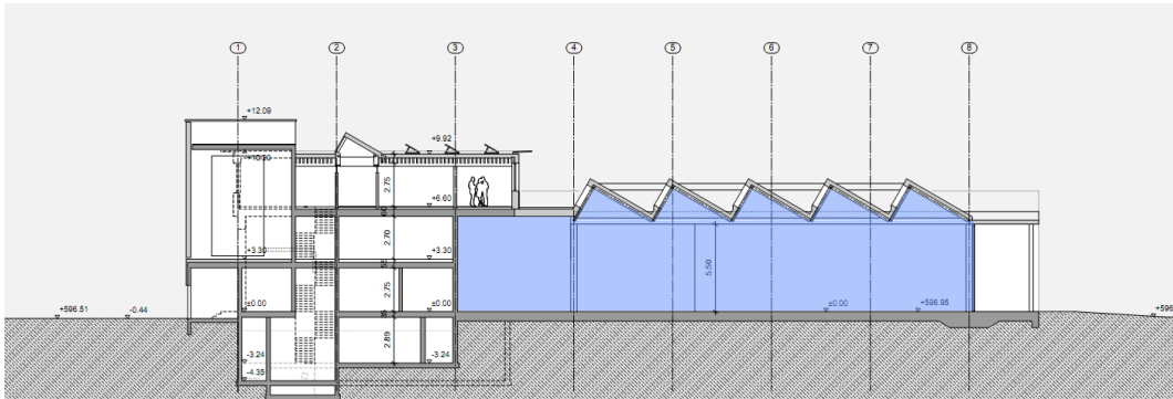
Schnitt B-B
