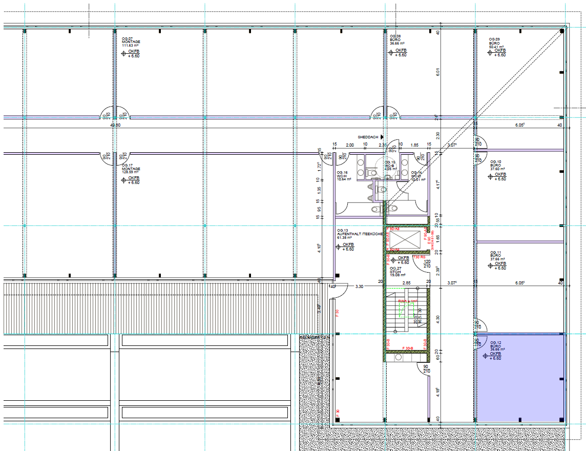
Grundriss Obergeschoss, östlicher Teil
