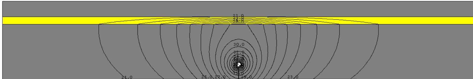
Wärmestromdichte innerhalb der aktivierten Stahlbetondecke
