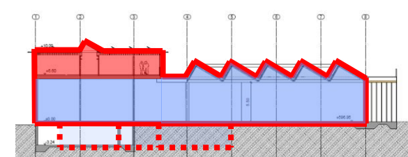
Schnitt B-B
