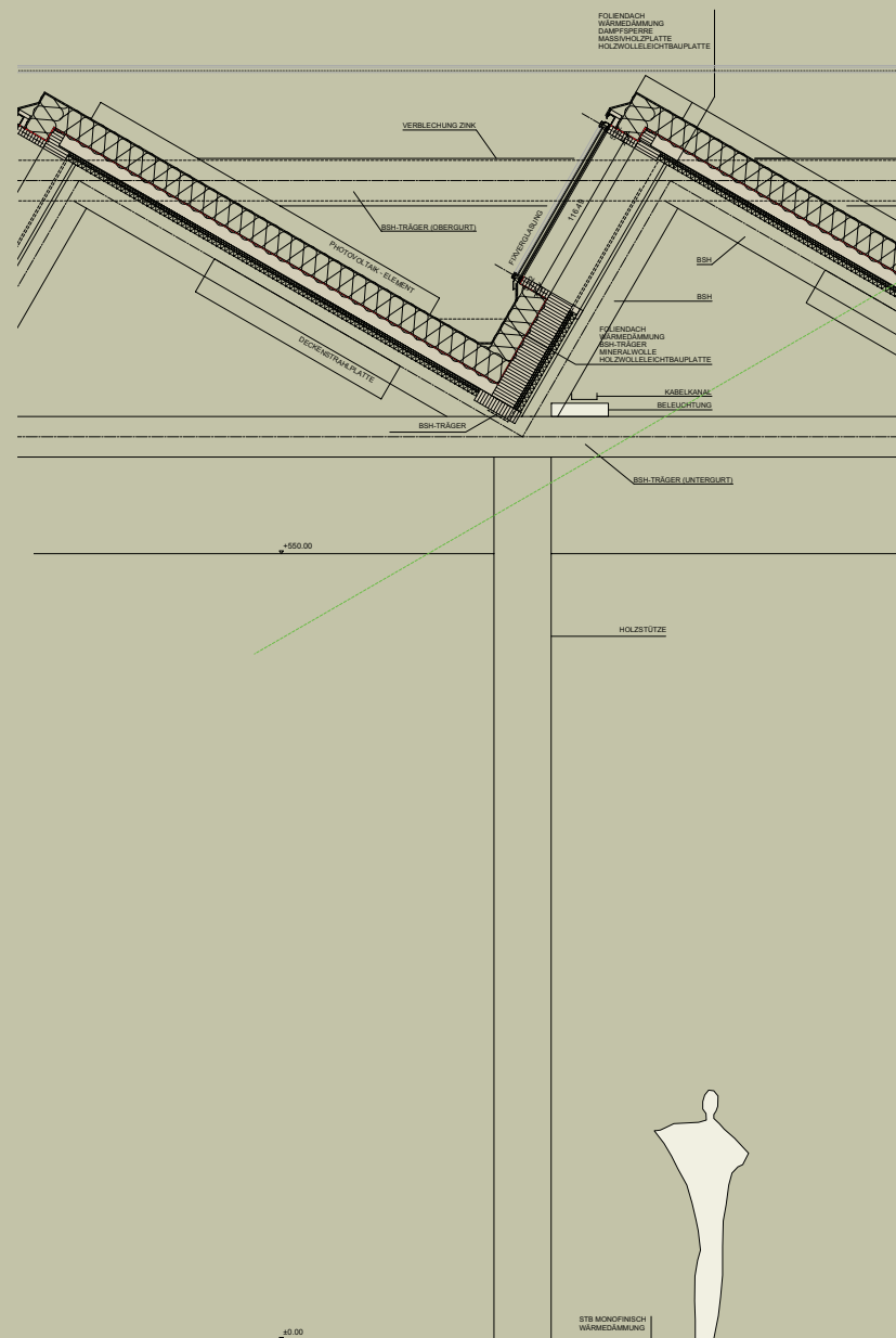
fassadenschnitt m1zu20
