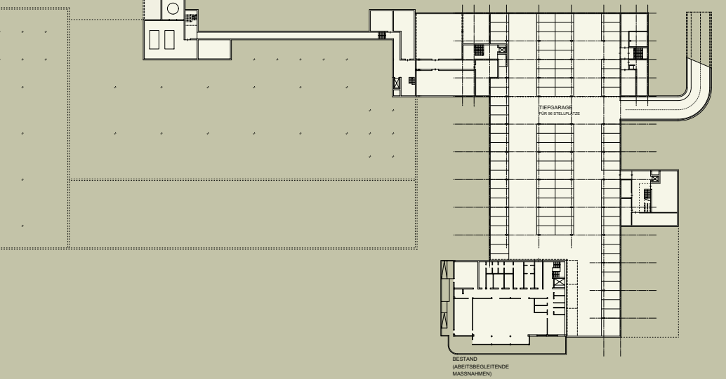
grundriss untergeschoss m1zu500
