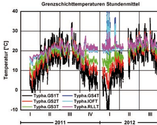
Bild 24: Verlauf der Grenzschnitttemperaturen als Stundenmittelwerte für den Zeitraum von Januar 2011 bis September 2012, Diagramm IBP
