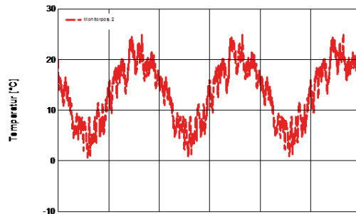
Bild 14: Zeitlicher Verlauf der Temperatur (oben) und der relativen Luftfeuchte (unten) zwischen Außenwand und Innendämmung bei einer Hinterströmung mit 1 m 3 /md, Diagramm IBP
