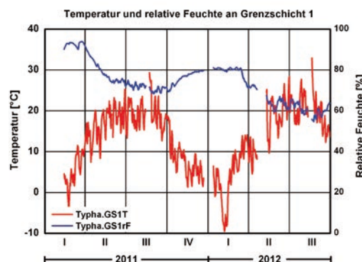
Bild 27: Verlauf der Temperatur und Feuchte an der Grenzschnitt 1, Diagramm IBP
