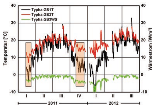
Bild 29: Hinter der Innendämmung (Grenzschicht 3) gemessener Wärmestrom zusammen mit dem Verlauf der Temperatur an der Grenzschicht 1 und 3. Die Balken zeigen Zeitbereiche, die für eine Beurteilung des Wärmewiderstandes geeignet sind, Diagramm IBP
