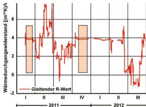
Bild 30: Aus den Messwerten (Bild 29) berechneter gleitender Wärmewiderstand (R-Wert). Die Balken zeigen Zeitbereiche, die für eine Beurteilung des Wärmewiderstandes geeignet sind, Diagramm IBP
