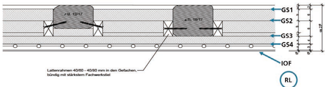
Bild 23: Schematischer Wandaufbau zusammen mit der Position der Grenzschichten bzw. Messstellen, Plangrundlage Architekturbüro Fritsch+KnodtKlug
