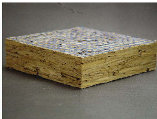
Bild 5: Chip-Board mit überwiegend waagrecht zur Plattenebene orientierten, größeren Partikel, zusammen mit den Materialkennwerten, Foto IBP
