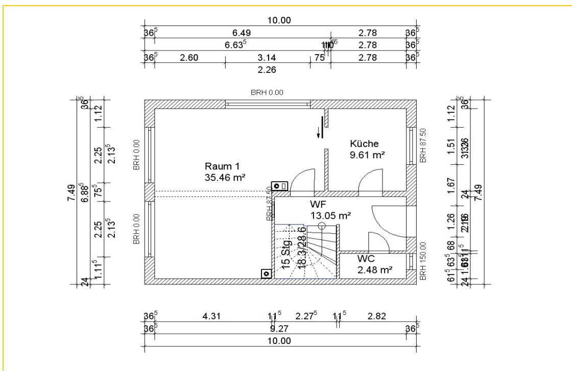
Abb. 7-5: Grundriss Doppelhaushälfte EG
