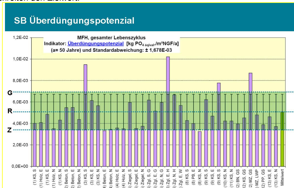
Abb. 9-24: Überdüngungspotenzial
