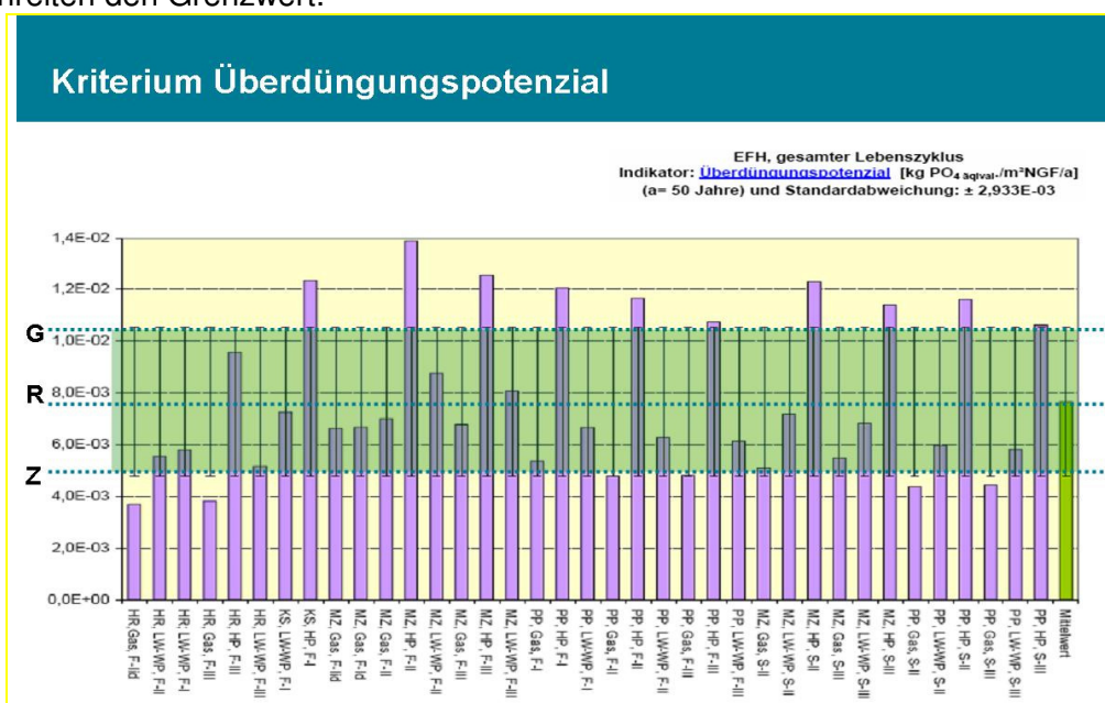
Abb. 9-5: Überdüngungspotenzial
