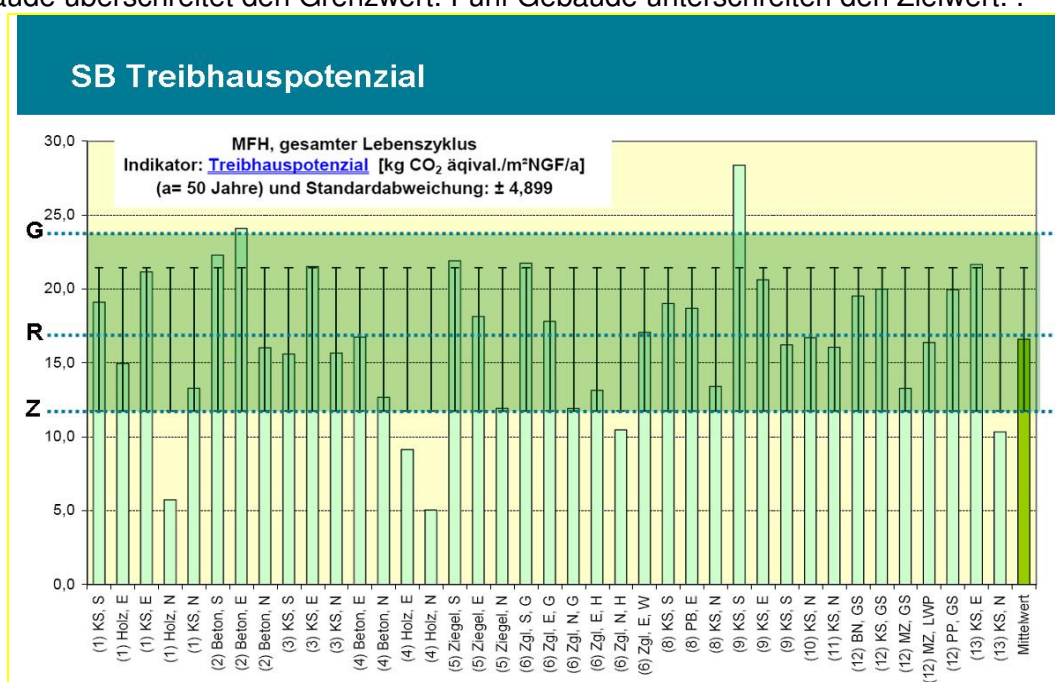
Abb. 9-20: Treibhauspotenzial
