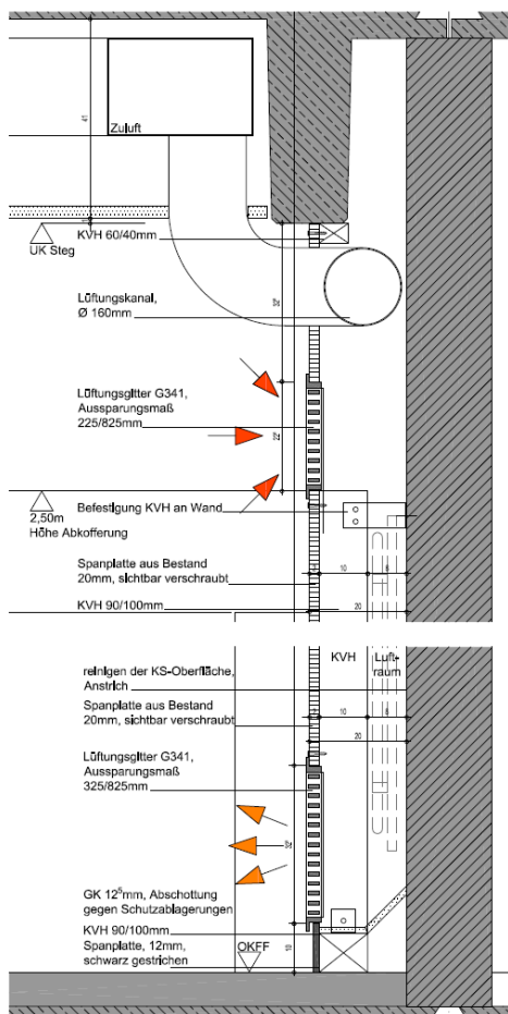
Abbildung 7-27: Technische Detailzeichnungen der Klimawand
