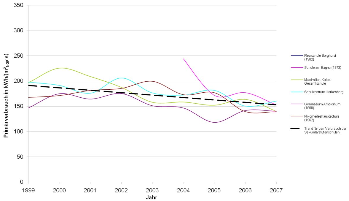
Abbildung 4-5: Primärenergieverbrauch in \text{kWh}/(\text{m}^2_{\text{NGF}}\cdot\text{a}) aller betrachteten Sekundärstufenschulen (witterungsbereinigt, Standort: MS/OS)
