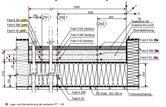
● Lage- und Kennzeichnung der verbauten PT - 100 Bild 5: Feld II, 20 cm Dämmung, 8 cm GTD M-Leicht sowie gestochener Grassoden.
