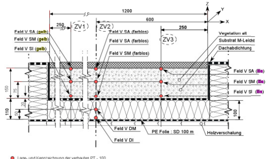
● Lage- und Kennzeichnung der verbauten PT - 100 Bild 8: Feld V, 10 cm Dämmung, 15 cm GTD M-Leicht sowie gestochener Grassoden.
