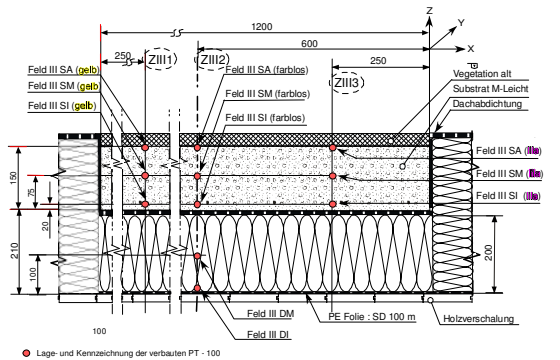
● Lage- und Kennzeichnung der verbauten PT - 100 Bild 6: Feld III, 20 cm Dämmung, 15 cm GTD M-Leicht sowie gestochener Grassoden.
