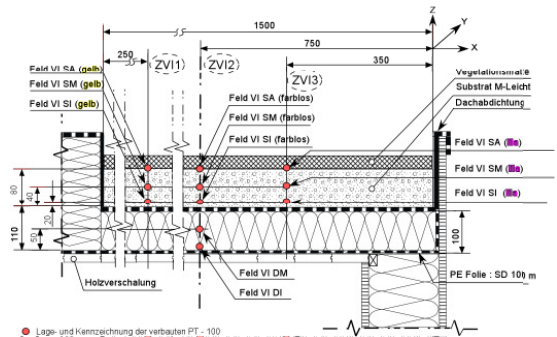
● Lage- und Kennzeichnung der verbauten PT - 100 Bild 9: Feld VI, 10 cm Dämmung 8 cm GTD M-Leicht sowie Vegetationsmatte SM/G.
