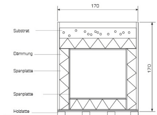
Bild 3: Schnitt durch den Versuchsstand.
