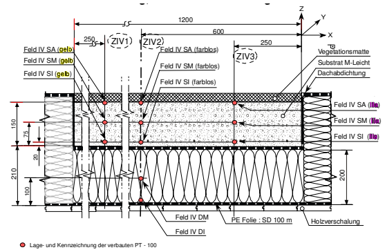
● Lage- und Kennzeichnung der verbauten PT - 100 Bild 7: Feld IV, 20 cm Dämmung, 15 cm GTD M-Leicht sowie Vegetationsmatte SKG/G.
