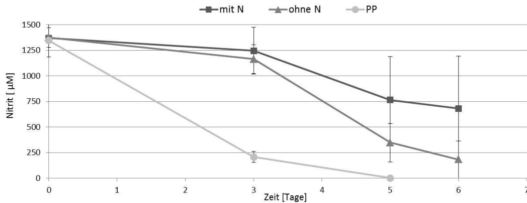
Abb. 10: Nitritoxidation durch angeheftete Zellen an Kunststofffolien aus vorhergegangenem Hemmtest (Abb. 9). „mit N“ = unter Stickstoffatmosphäre beschichtet, PP = Kontrollfolie ohne Beschichtung.
