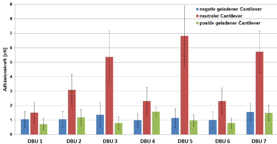
Abb. 6: Interaktionen zwischen negativ (blau), neutral (rot) und positiv (grün) geladenen Cantilevern und den jeweiligen Oberflächen der PP-Folien. Die Fehlerbalken zeigen die Standardabweichung, n=3, Mittelwerte errechnet aus je 3750 Einzelmessungen
