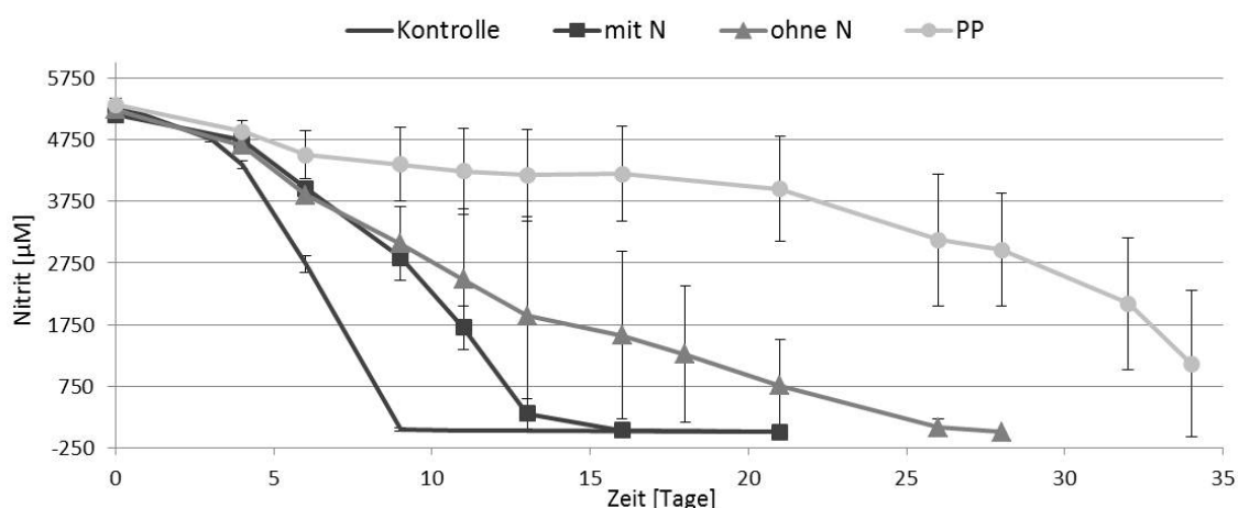
Abb.9: Oxidation von Nitrit in Medien mit PP- Folien und im Kontrollmedium ohne Kunststofffolien. „mit N“ = unter Stickstoffatmosphäre beschichtet, PP = Kontrollfolie ohne Beschichtung.
