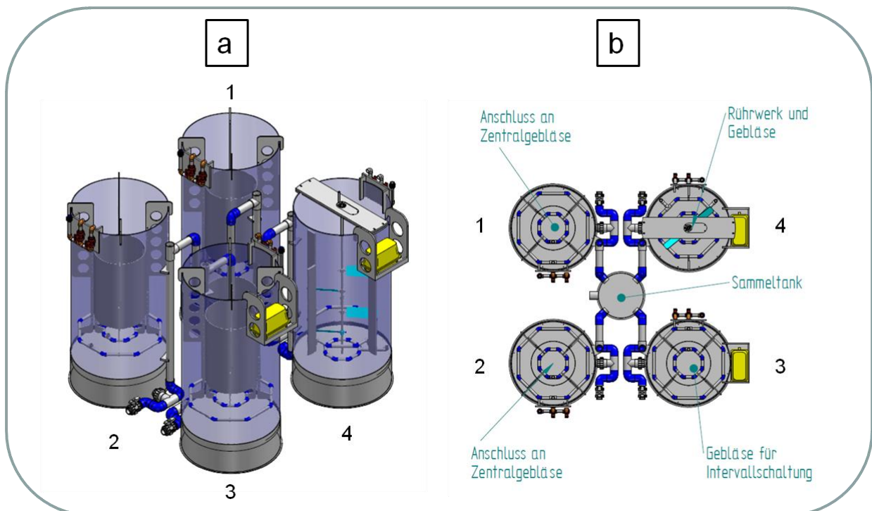
Abb. 18: Schematische Darstellung (© Spranger Kunststoffe) der vier Versuchsbiofilterreaktoren mit unterschiedlichen Belüftungsverfahren. a: Seitenansicht; b: Aufsicht. 1: Konventionelle Belüftung (Kontrolle); 2: Reduzierte Einblastiefe; 3: Intervall-Belüftung; 4: Mechanische Durchmischung (Rührer).
