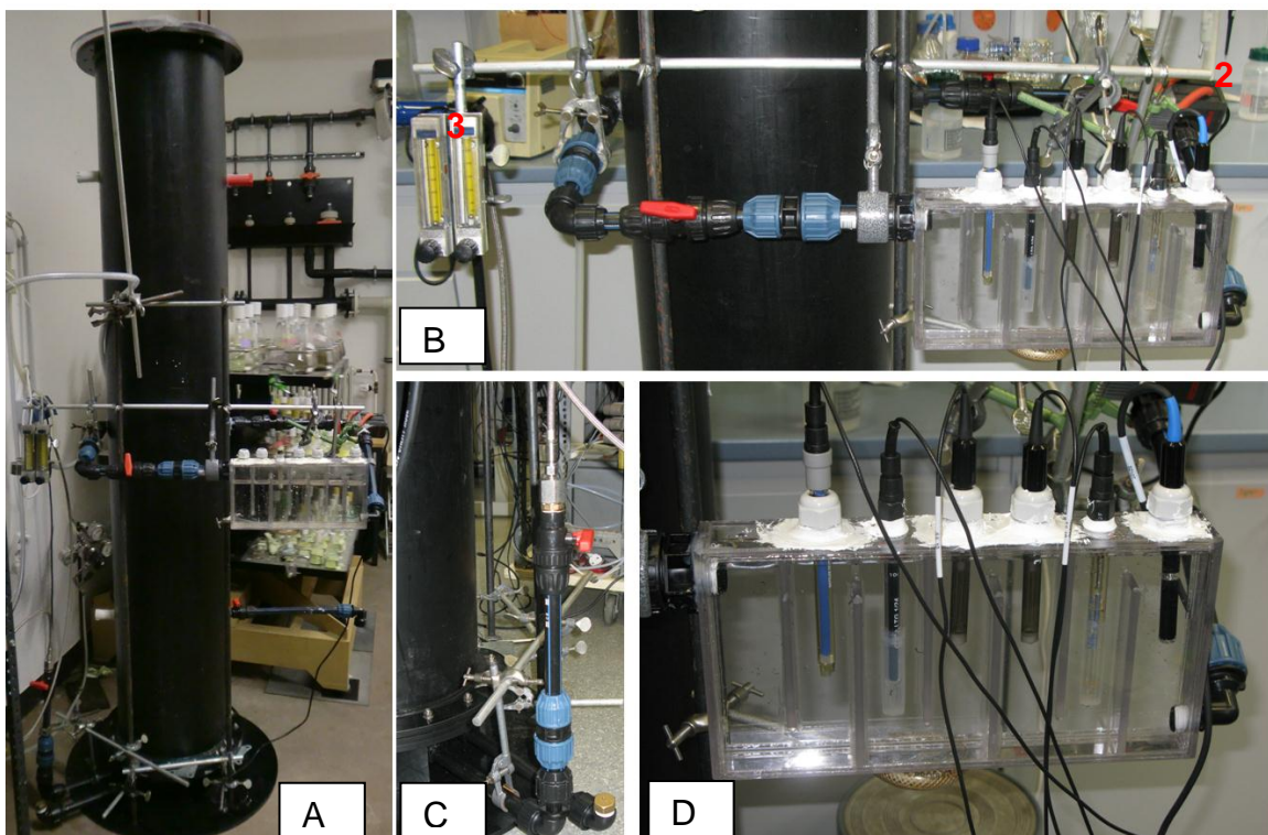
Abb. 23: Darstellung des Bioreaktors mit Online-Monitoring. (A) gesamter Bioreaktor, (B) links Durchflussregler der Druckluft und rechts Bypass mit Durchflusskammer und Elektroden für die Online-Überwachung, (C) Druckluftanschluß und (D) Detailaufnahme der Durchflusskammer mit Elektroden
