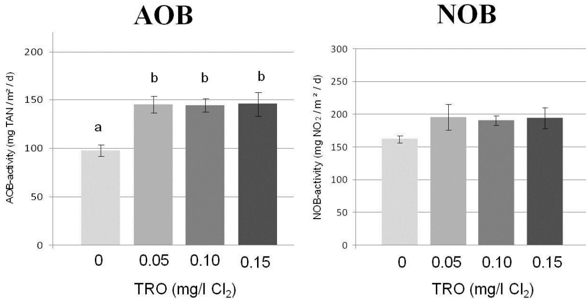
Abb. 16: Aktivität von Ammoniak oxidierenden Bakterien (AOB) und Nitrit oxidierenden Bakterien (NOB) in Abhängigkeit von der Restoxidantien-Konzentration (TRO) nach 21-tägiger Exposition. Unterschiedliche Buchstaben kennzeichnen signifikante Unterschiede zwischen den Versuchsgruppen.
