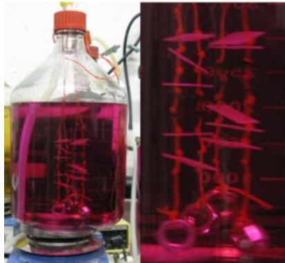
Abb. 1: Versuchsaufbau zur Anheftung von Referenzorganismen an die DBU Folien.
