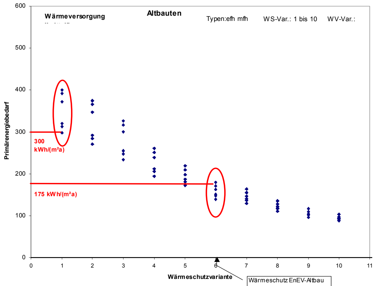
Abbildung 4-1: Primärenergiekennwert für unterschiedliche Varianten des Wärmeschutz bei mittlerer Effizienz des Heizungssystems für Ein- und Mehrfamilienhäuser
