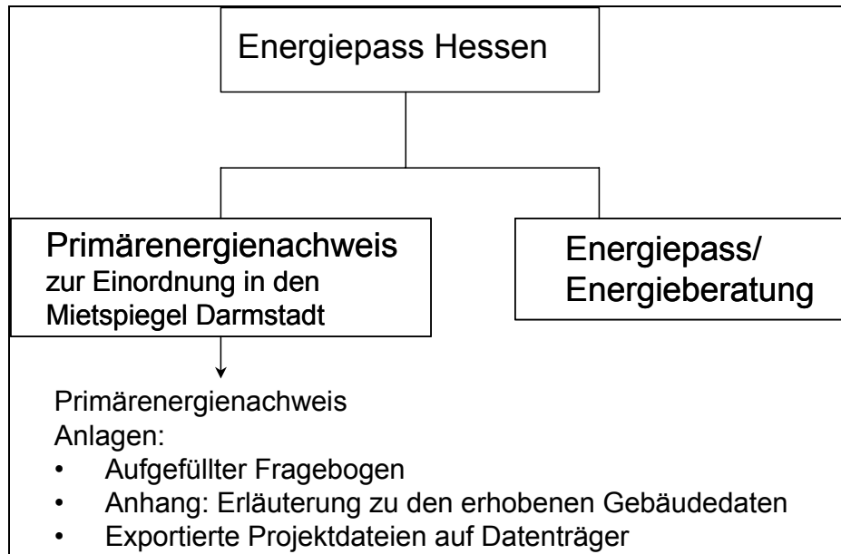
Abbildung 7-1: Konzept zum Nachweis des Primärenergiekennwerts für die Einordnung in den Mietspiegel Darmstadt
