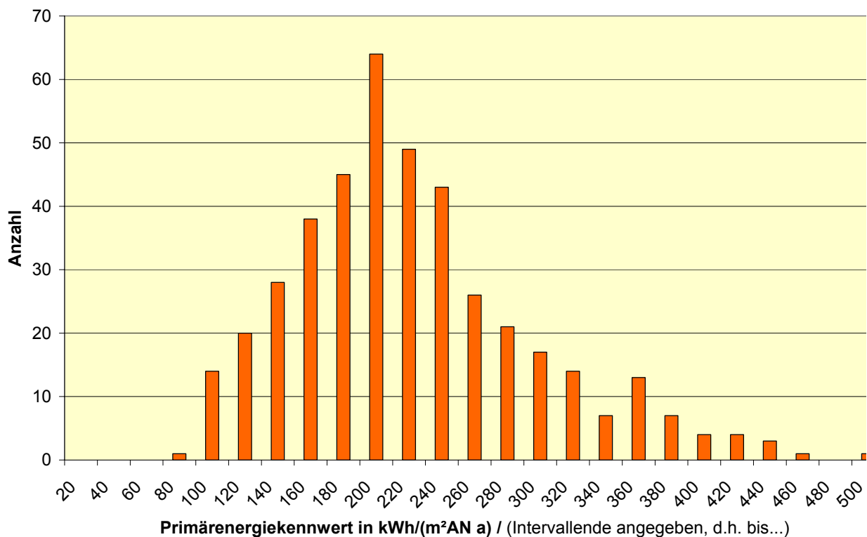
Abbildung 3-2: Häufigkeitsverteilung des Primärenergiekennwerts
