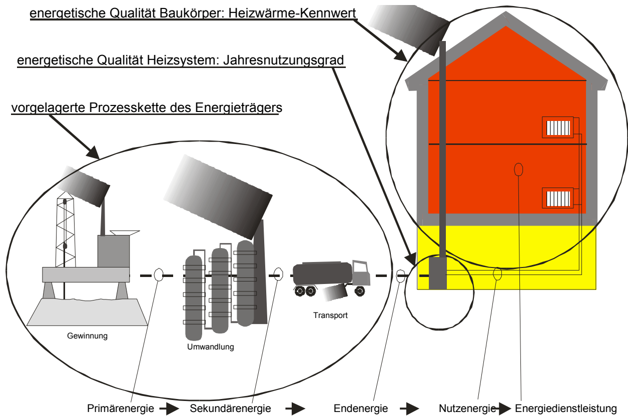
Abbildung 2-2: Bilanzgrenze des Primärenergiekennwerts
